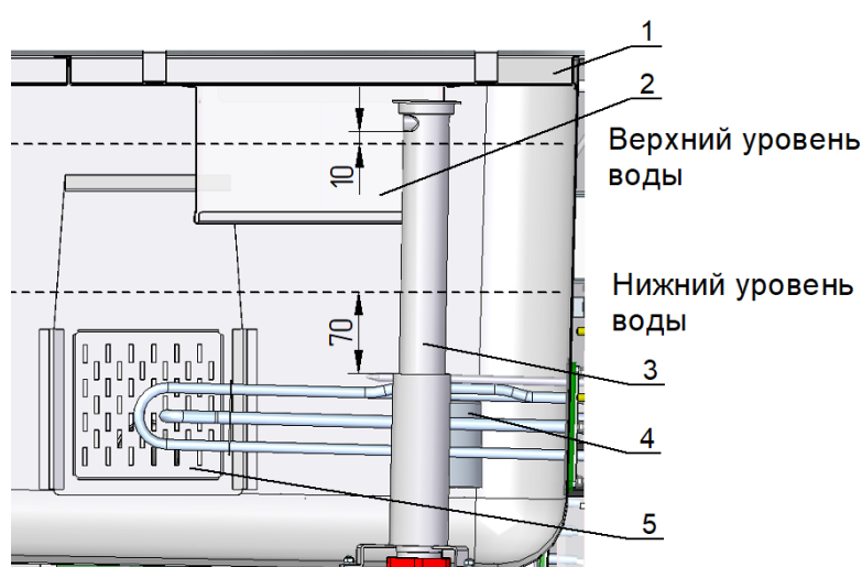
Рис. 4. Верхний и нижний уровни воды в ванне
