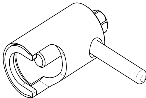
Рис. 9. Съемник крыльчатки.
